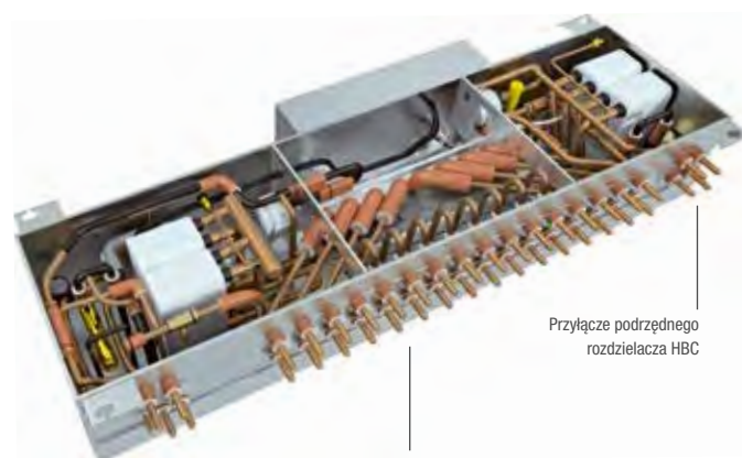
Przylączy przewodów zasilających i powrotnych do systemu wodociągowego; dostępne są wersje z 8 lub 16 przylączami.
