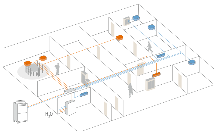
Zasada działania ekonomicznego systemu 2-rurowego z odzyskiem ciepła do jednoczesnego chłodzenia i grzania.
